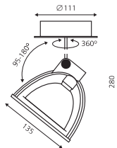
0015760 Einzelleuchte, Nickel für Aufbau oder Teileinbau integrierter Trafo 240/12V 50W singular luminary, nickel, for building up or partial installation, integrated trafo 240/12V 50W
